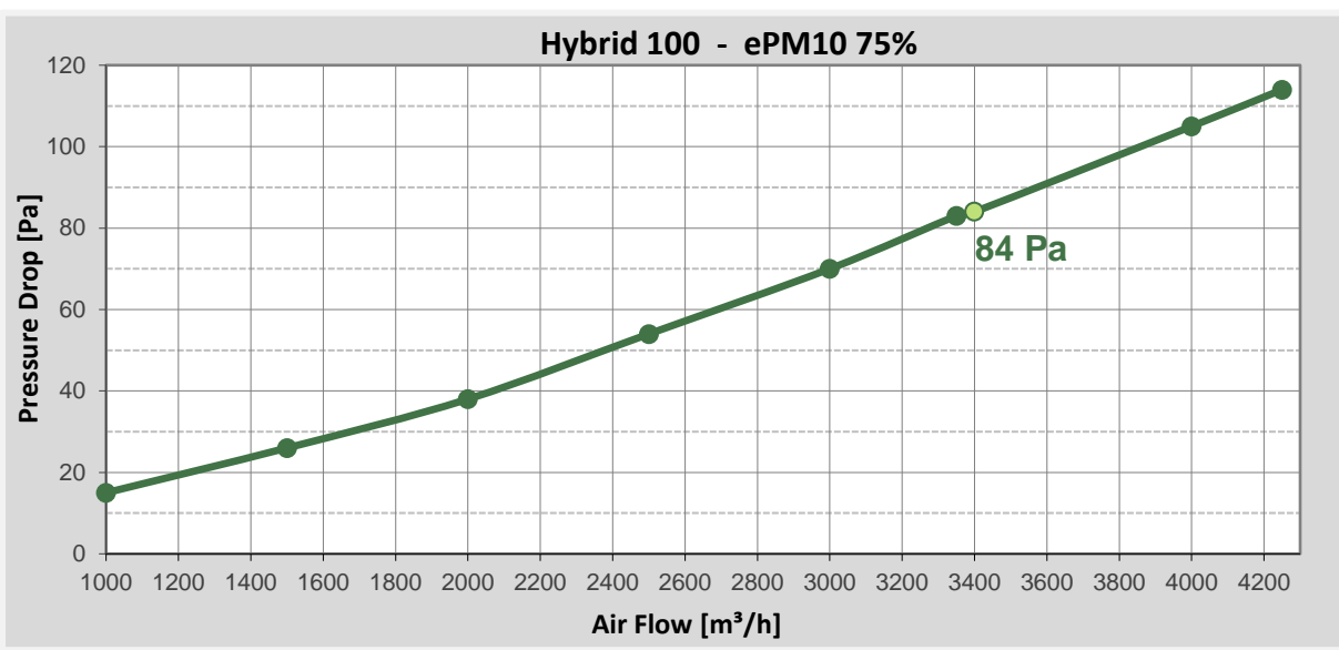
Panelfilter 593x593x96 mm @ 3400 m³/h
