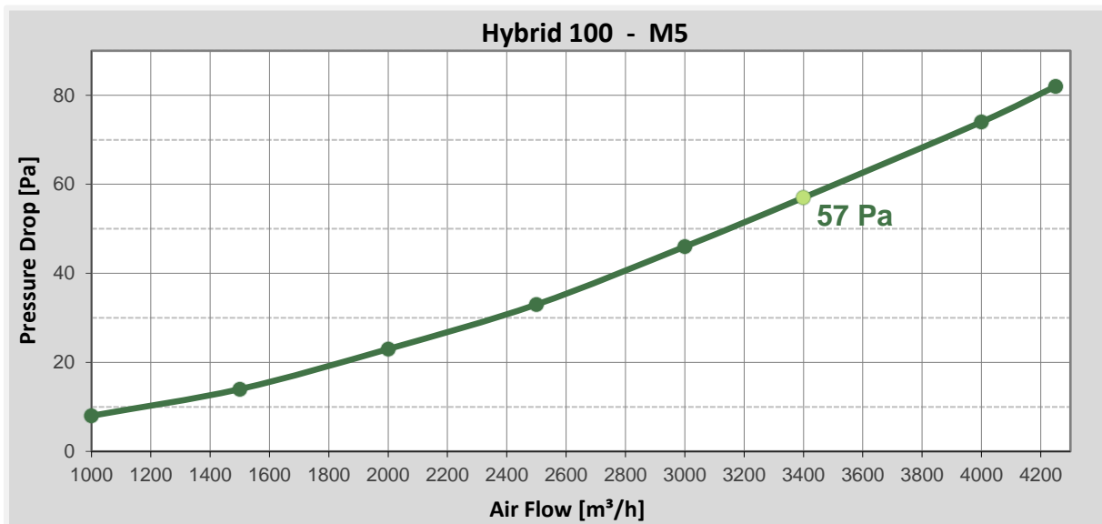
Panelfilter 593x593x96 mm @ 3400 m³/h
